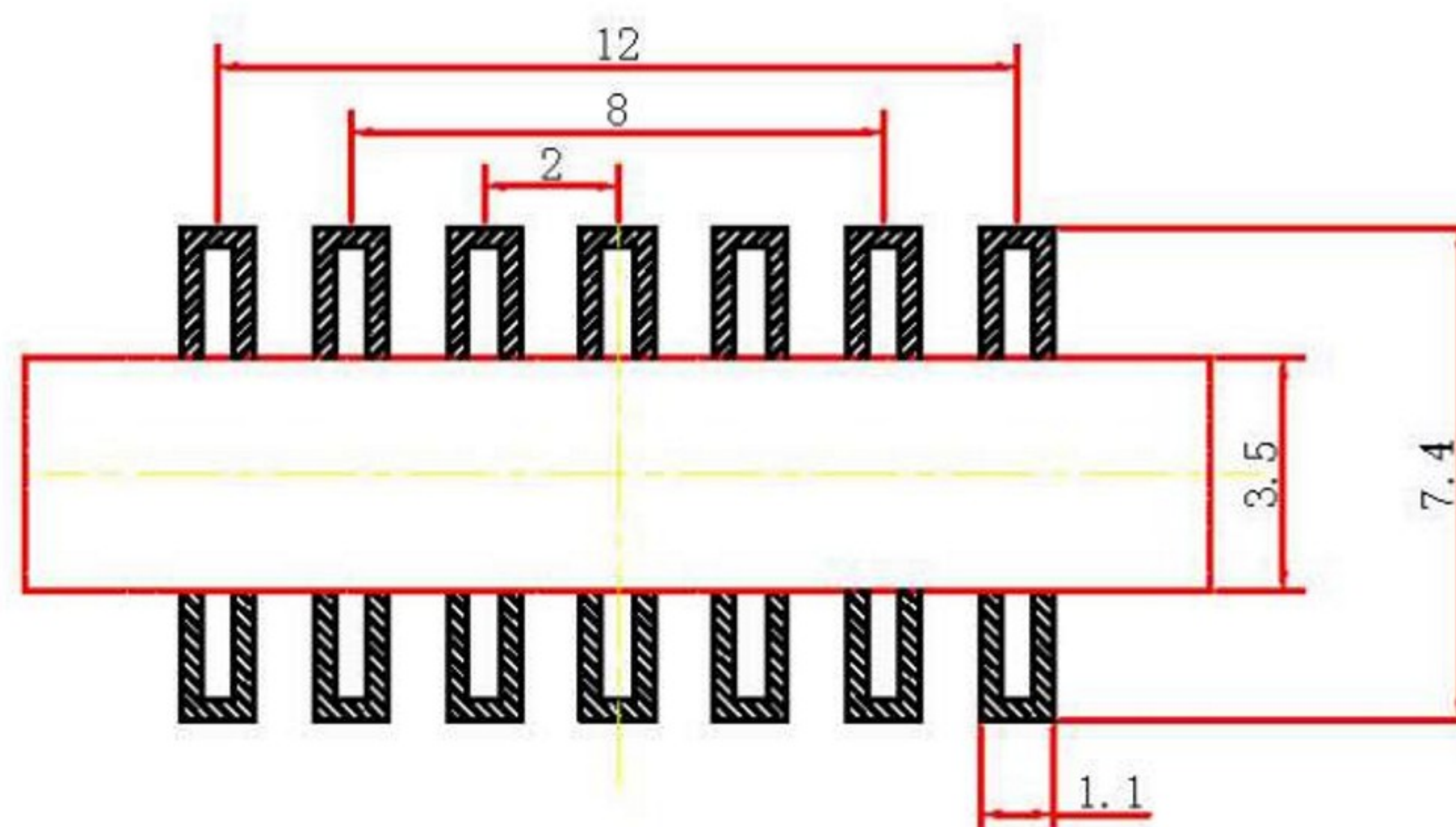
PCB板位置尺寸
