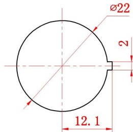
安装尺寸
