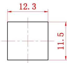
安装尺寸
