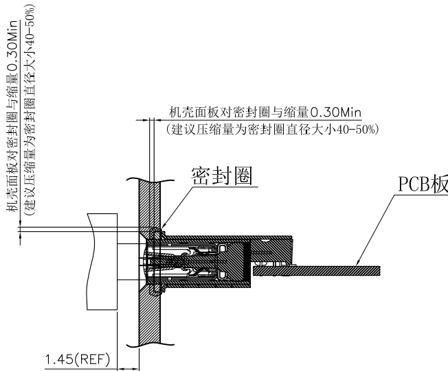
组装机壳后公母头对插示意图
