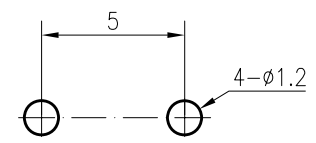
PCB线路板安装图(±0.1)
