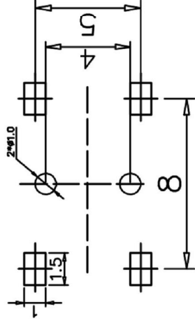
安装孔位图
