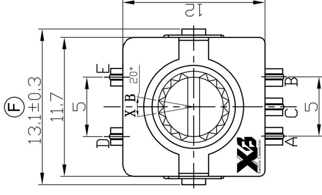
(SW01) ENCODER
