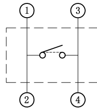
电路图：常开式 (N.O) 1个电路1个接点 端子排列（自A方向看）
