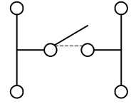
电路图：常开式(N.O) 1个电路1个接点 端子排列（自A方向看）
