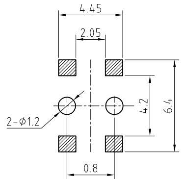
印制电路板及焊接安装孔参考图 （自A方向看）
