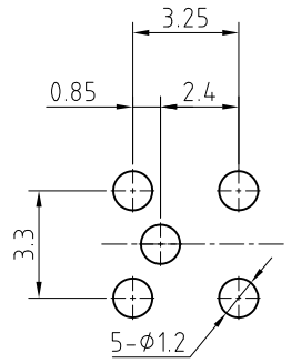
印制电路板及焊接安装孔参考图 （自A方向看）
